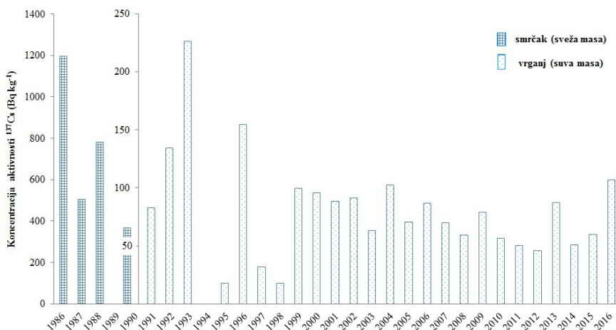
Slika 1. Godišnje srednje vrednosti koncentracija aktivnosti ^{137}\text{Cs} u uzorcima gljiva za period 1986-2016. (smrčak (sveža masa) (1986-1990) i vrganj (suva masa) (1991-2016))
