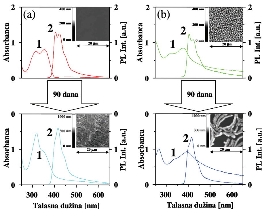
Slika 5. Apsorpcioni i PL spektri i AFM slike deponovanih TPD filmova, evaporisanih 3 min, snimljeni na različitim udaljenostima od nulte tačke: a) 1,0 i b) 31,0 mm, neposredno nakon evaporacije i posle 90 dana. (1 – apsorpcioni, 2 – PL spektar).
