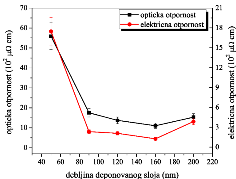
Slika 6.44. Poređenje optičke i električne otpornosti tankih slojeva nikla mjenjenih spektroskopskom elipsometrijom i metodom četiri tačke
