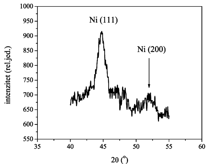
Slika 6.62. Difraktogram snimljen za uzorak nikla debljine 290 nm
