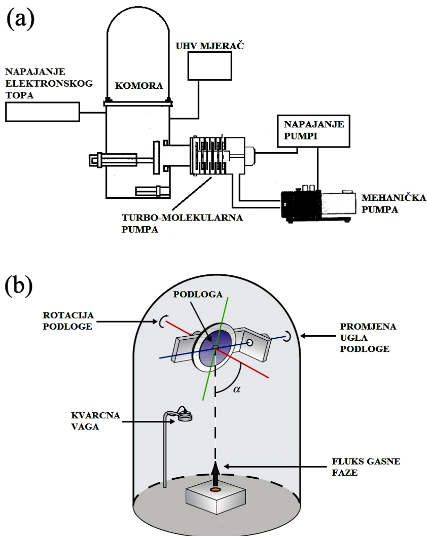
Slika 5.1. Šematski prikaz: (a) uređaja za deponovanje i (b) sistema za isparavanje materijala
