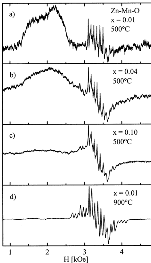
Slika 6. EPR spektri na sobnoj temperaturi za Zn-Mn-O: (a) x = 0,01 termički tretiran na 500\text{ }^{\circ}\text{C} , (b) x = 0,04 termički tretiran na 500\text{ }^{\circ}\text{C} , (c) x = 0,10 termički tretiran na 500\text{ }^{\circ}\text{C} , (d) x = 0,01 termički tretiran na 900\text{ }^{\circ}\text{C} .
