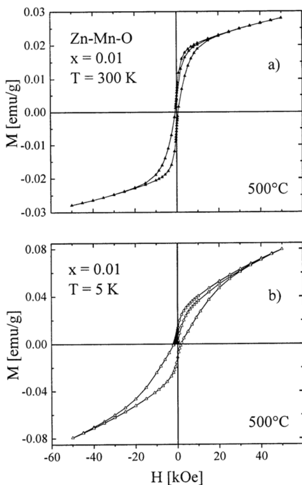
Slika 3. Magnetizacija u funkciji magnetnog polja na temperaturi (a) 300 K, (b) 5 K, za Zn-Mn-O, x = 0,01 termički tretiran na 500 °C.
