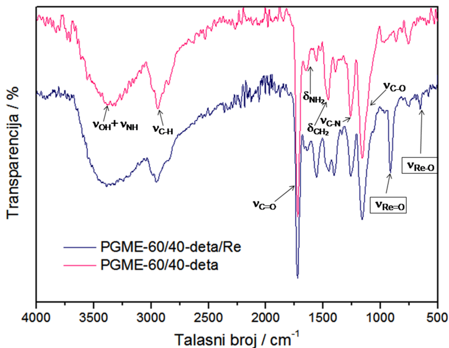
Slika 4.7.2. FTIR-ATR spektri uzoraka PGME-60/40-deta i PGME-60/40-deta/Re.
