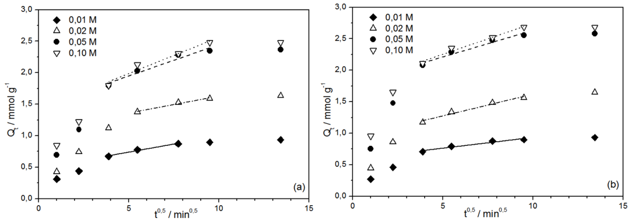
Slika 4.5.7. Grafički prikaz linearizovanog oblika kinetičkog modela unutarčestične difuzije za sorpciju Cr(VI) pomoću (a) PGME-60/40-deta i (b) PGME-80/20-deta za navedene početne koncentracije rastvora Cr(VI).
