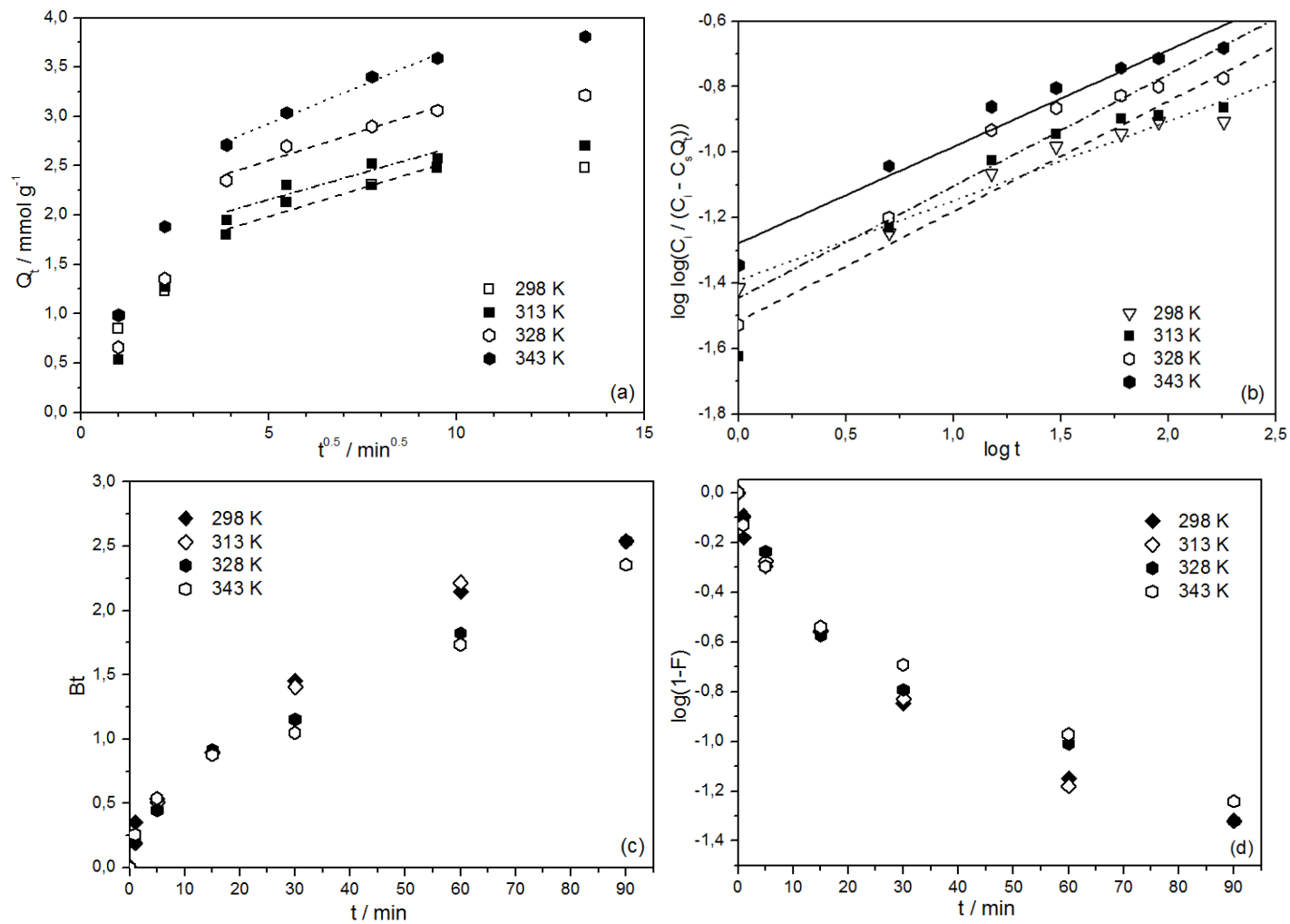
Slika 4.5.19. Grafički prikaz linearizovanih oblika kinetičkih modela za sorpciju Cr(VI) pomoću PGME-60/40-deta: (a) unutarčestične difuzije, (b) Bangamovog, (c) Bojdovog i (d) Mek Kejevog modela za navedene temperature.
