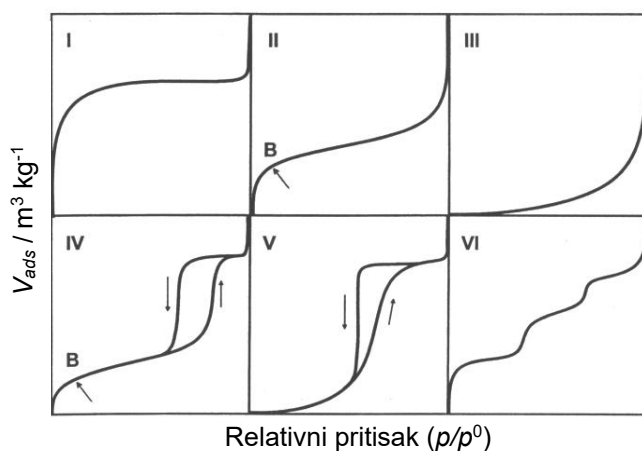
Slika 2.3.3. Tipovi adsorpciono–desorpcionih izotermi [35].
