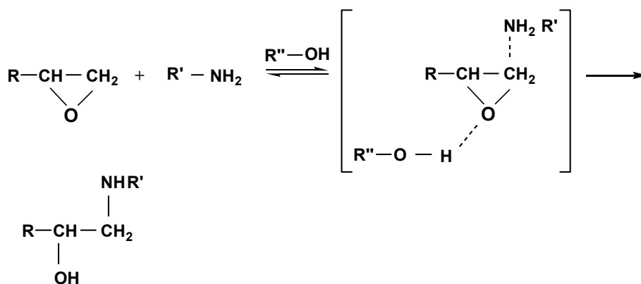
Slika 2.5.2. Mehanizam reakcije epoksidne grupe sa amino/amidnim jedinjenjima [86].
