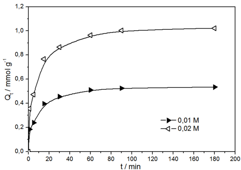
Slika 4.5.14. Zavisnost kapaciteta sorpcije PGME-60/40-deta od vremena kontakta za C_i = 0,01 i 0,02 \text{ mol dm}^{-3} rastvora Cr(VI) ( \text{pH} = 3,8 ).
