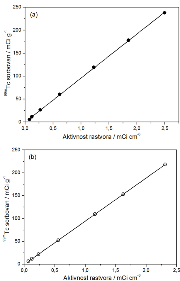
Slika 4.6.4. Grafik zavisnosti količine sorbovanog ^{99m}\text{Tc}(\text{VII}) na (a) PGME-60/40-deta i (b) PGME-80/20-deta od ravnotežne aktivnosti rastvora (pH = 3,0).
