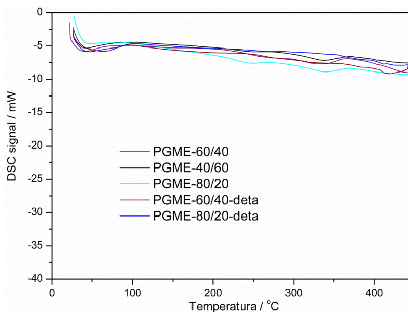
Slika 4.3.9. DSC krive za uzorke PGME sa različitim udelom EGDMA i naznačene amino-funkcionalizovane uzorke.
