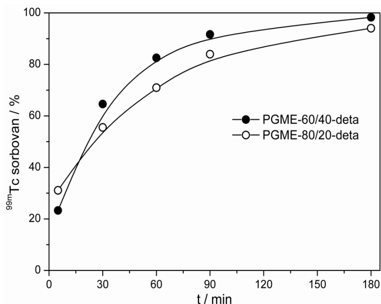
Slika 4.6.1. Zavisnost procenta uklanjanja ^{99m}\text{TcO}_4^- pomoću PGME-60/40-deta i PGME-80/20-deta od vremena kontakta.
