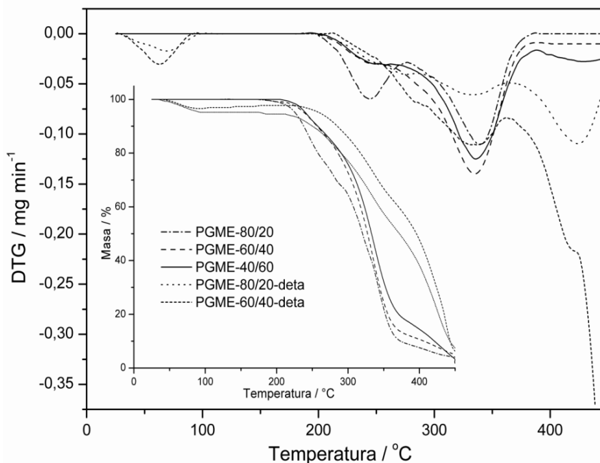
Slika 4.3.8. DTG i TG termogrami za uzorke PGME sa različitim udjelom EGDMA i naznačene amino-funkcionalizovane uzorke (brzina zagrevanja 10\text{ }^{\circ}\text{C min}^{-1} , protok helijuma 30\text{ cm}^3\text{ min}^{-1} , temperaturni interval 25\text{--}450\text{ }^{\circ}\text{C} ( 298\text{--}723\text{ K} )).
